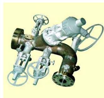
4500psi-5"/3" ジャケット付き 洗浄弁 3 台 (3"+2") 付き
